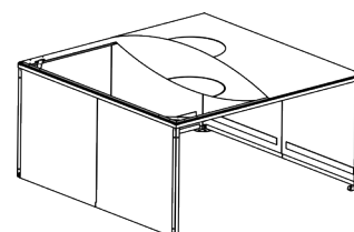
Cumulus
